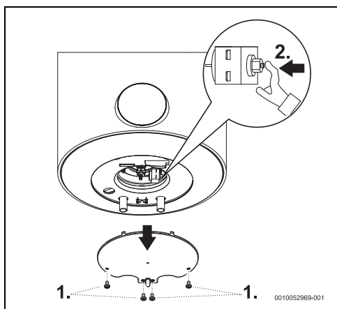
10. ábra Biztonsági hőmérséklet-határoló
