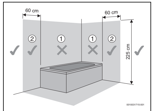
5. ábra Védőzóna
