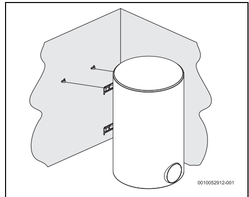
Sl.7 Navpična montaža (pritrditev na steno)
