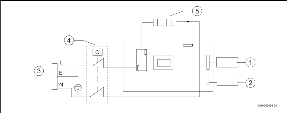
Sl.11 Shema ožičenja
