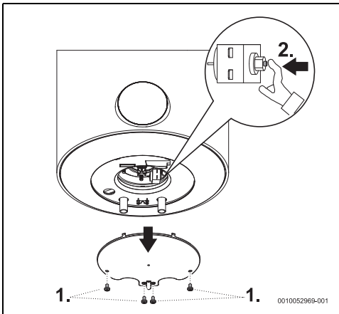
Сл. 10 Безбедносен термостат
