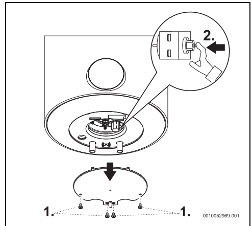
Sl. 10 Varnostni termostat
