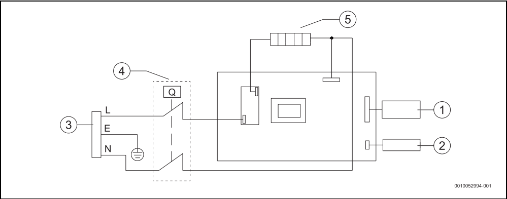
Сл. 11 Дијаграм на поврзување
