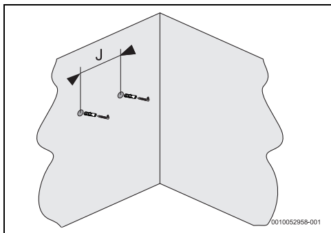
Сл. 6 Завртки за прицврстување
