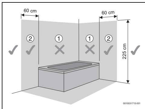
Rys. 5 Strefa ochronna
