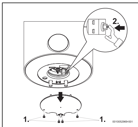
Rys. 10 Termostat zabezpieczający
