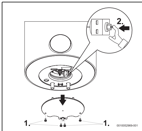
sl. 10 Sigurnosni termostat
