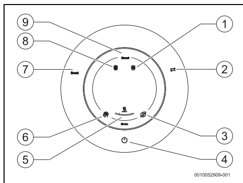
Rys. 4 Panel sterowania
