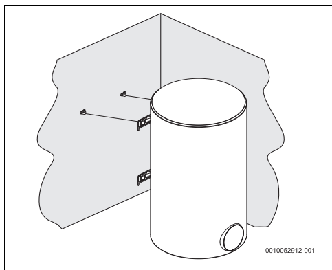
Fig. 7 Instalare verticală (montare pe perete)
