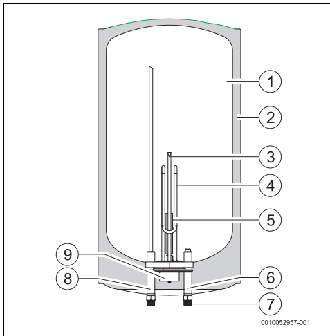
3. ábra A készülék komponentjei
