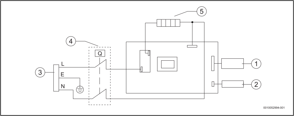
sl. 11 Šema povezivanja
