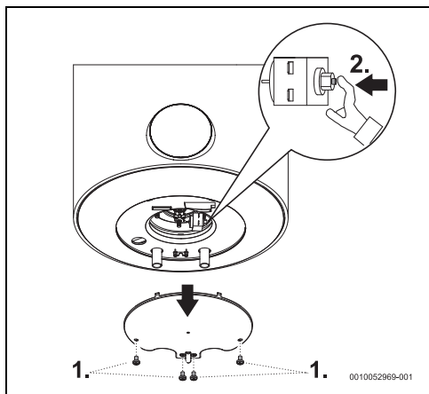
Fig. 10 Termostat de siguranță
