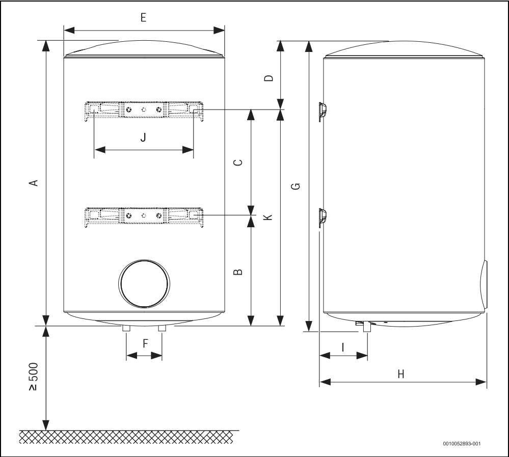
Sl.2 Mere v mm (pritrditev na steno, navpična montaža)
