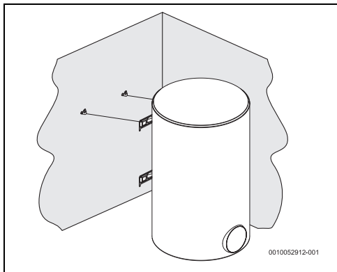
7. ábra Fügőleges telepítés (falra szerelés)
