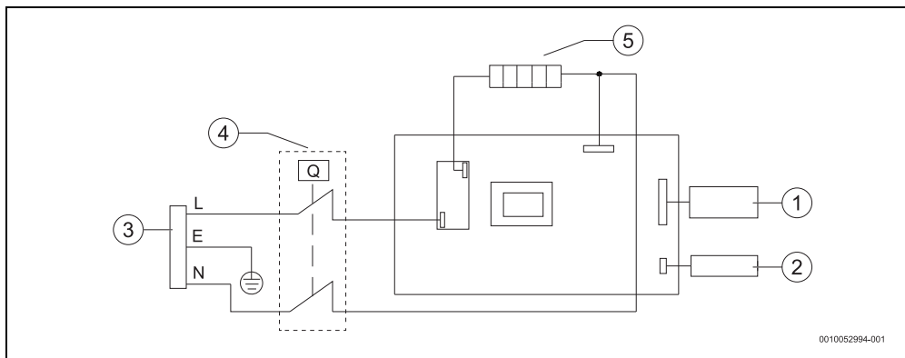
11. ábra Csatlakoztatási rajz
