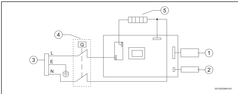
Rys. 11 Schemat połączeń
