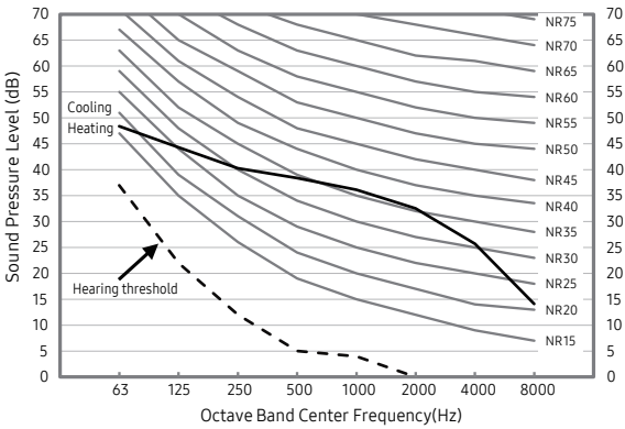
1) AE050CXYBEK/EU
