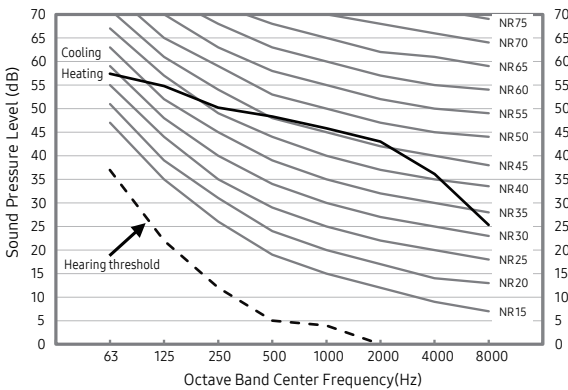
4) AE160CXYBEK/EU
