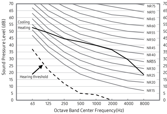
2) AE080CXYBEK/EU
