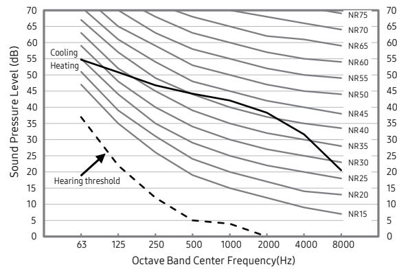
6) AE120CXYBGK/EU
