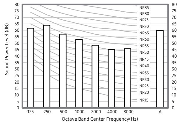
6) AE120CXYBGK/EU
