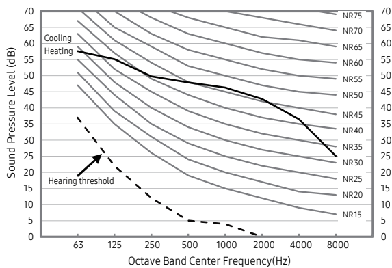
7) AE160CXYBGK/EU
