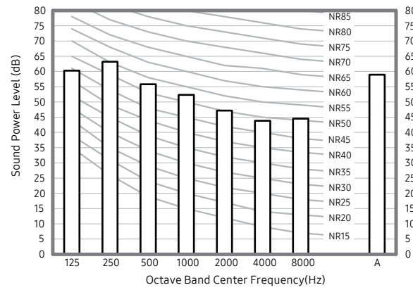
2) AE080CXYBEK/EU
