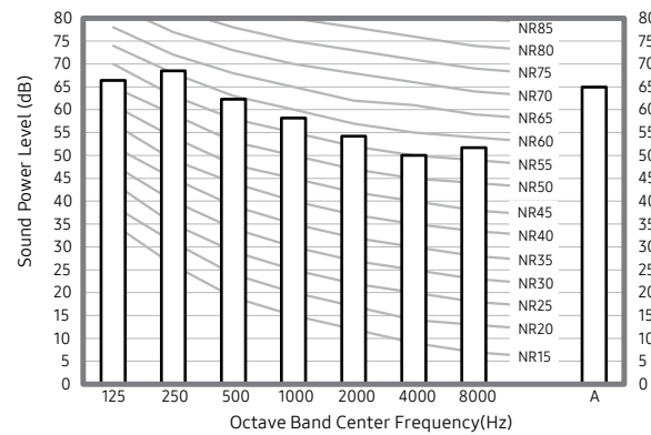
4) AE160CXYBEK/EU
