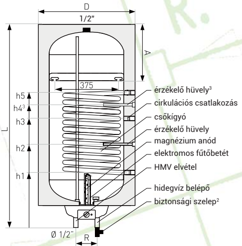
Plus típusú vízmelegítő rajza
