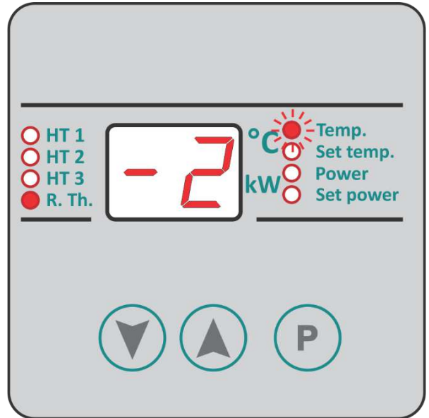
22. ábra: A kazán működésének letiltása fagyveszély miatt
