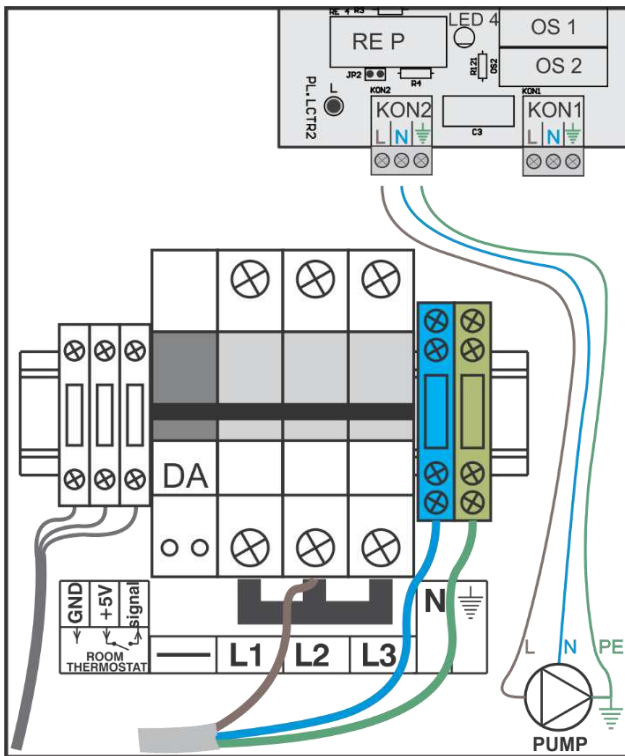
8. ábra: NOARK biztosítékok A kazán csatlakoztatási vázlatja Egy fázisú csatlakozás esetén Tápellátás – kizárólag 6 kW és 9 kW-os készülék esetében
