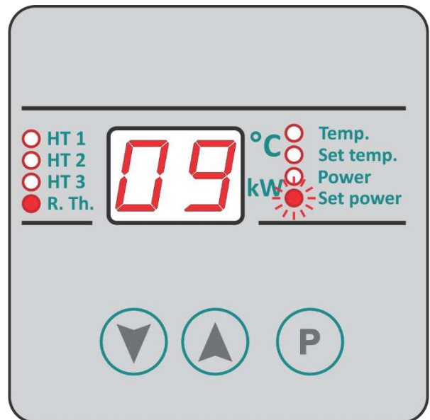
17. ábra: Kazán teljesítmény beállítás
