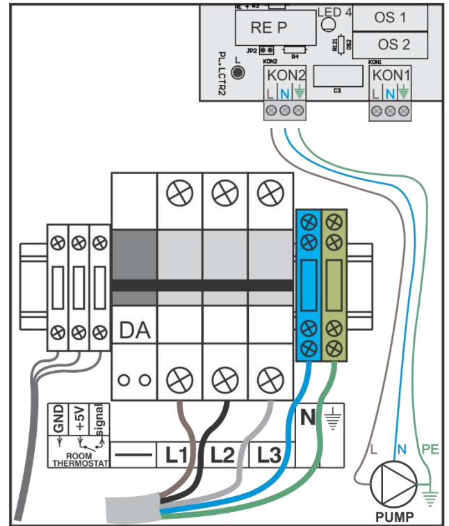
9. ábra: NOARK biztosítékok A kazán csatlakoztatási vázlatja három fázisú tápellátáshoz
